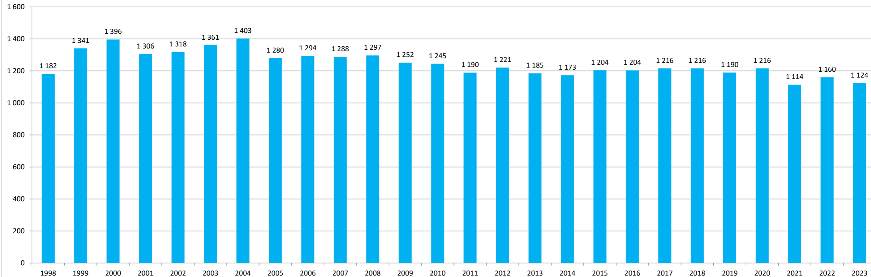
Voda určená k realizaci v tis. m 3 - provoz vodovodů Lanškroun
