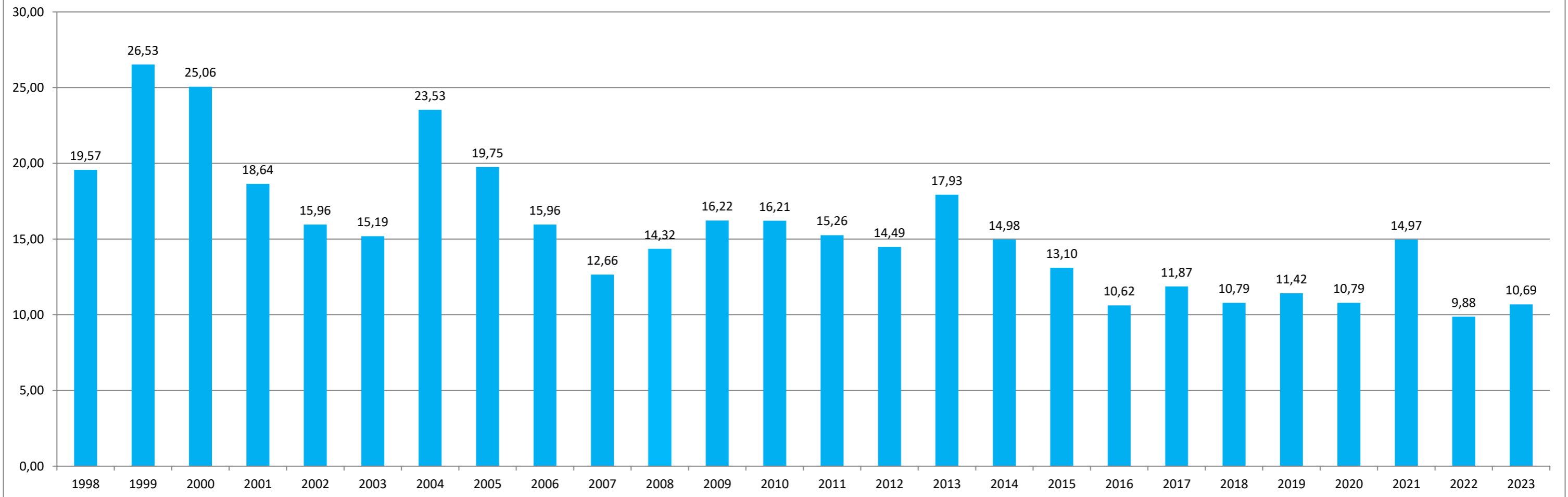
Ztráty ve vodovodní síti v % - provoz vodovodů Letohrad
