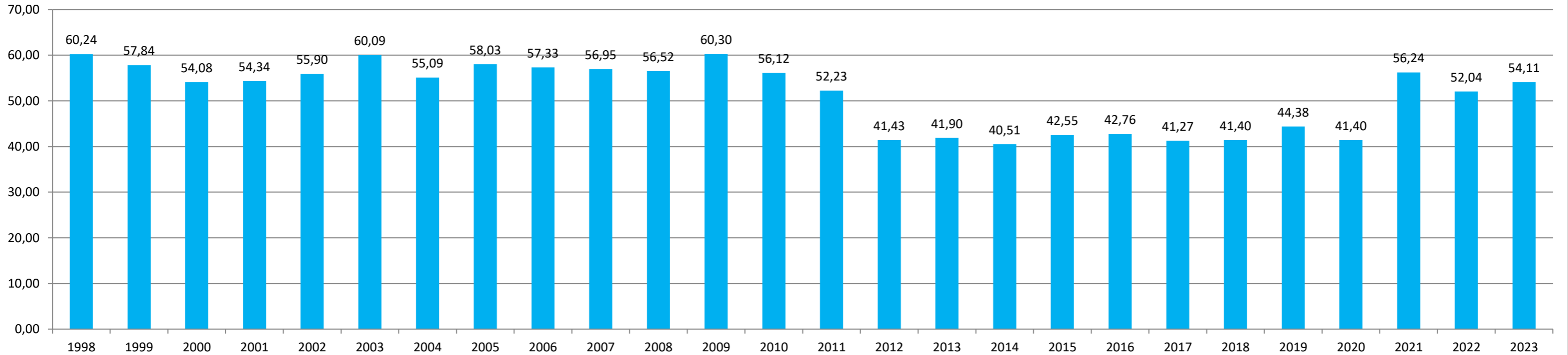
Podíl vody fakturované obyvatelstvu v % - provoz vodovodů Lanškroun
